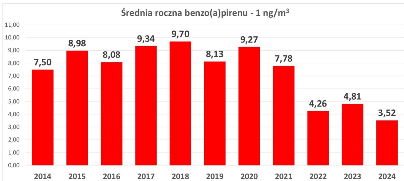
Wykres nr 10. Średnia roczna benzo(a)pirenu – 1 \text{ng}/\text{m}^3 w latach 2014-2024
