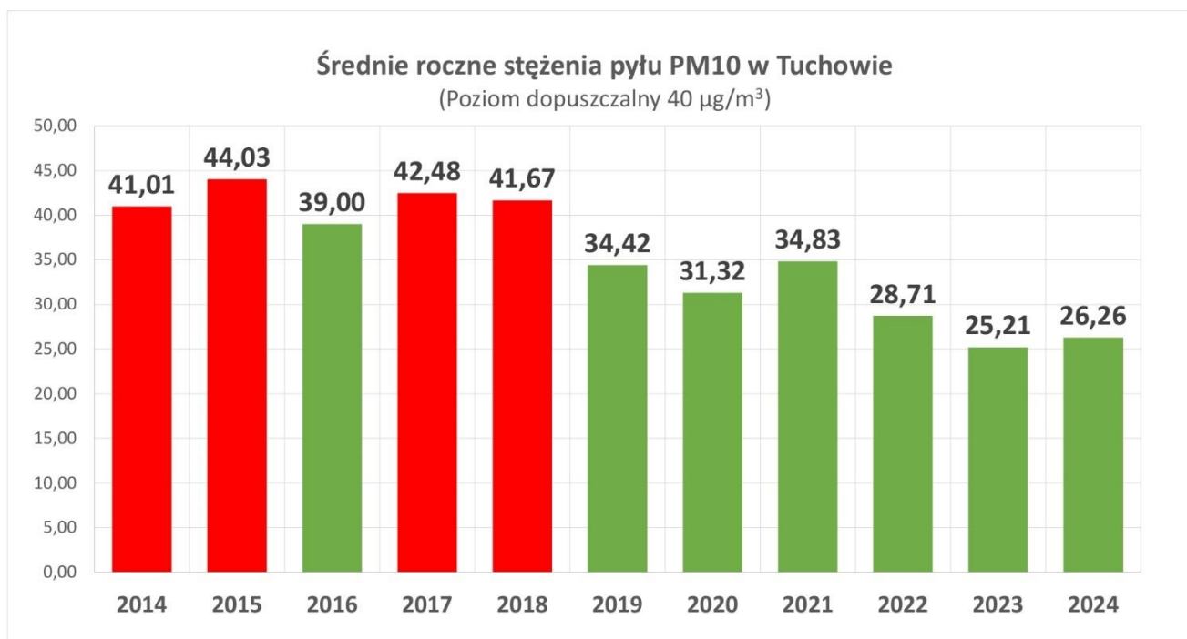
Wykres nr 9. Średnio roczne stężenia pyłu PM10 w latach 2014-2023 (poziom dopuszczalny 40 \mu\text{g}/\text{m}^3 )
