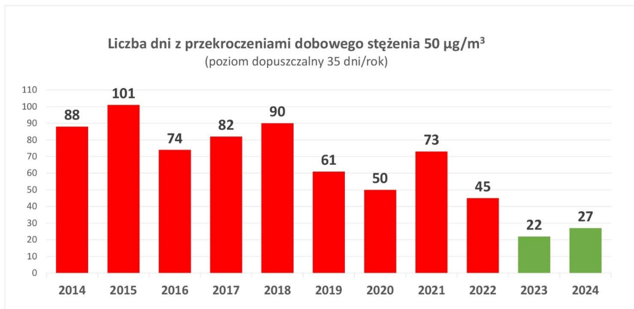
Wykres nr 11. Liczba dni z przekroczeniami dobowego stężenia pyłu PM 10 (50 µg/m 3 ) w latach 2014-2024 (poziom dopuszczalny 35 dni/rok)
